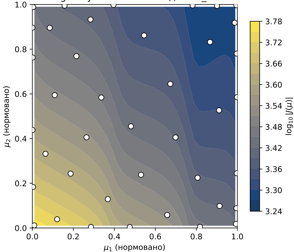
P-greedy: 40 точок на задачі rd_2d
